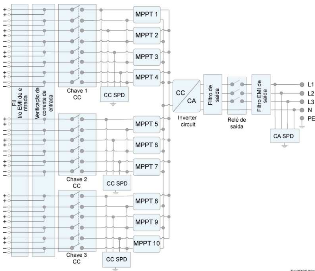
Figura 2-10 Diagrama esquemático
