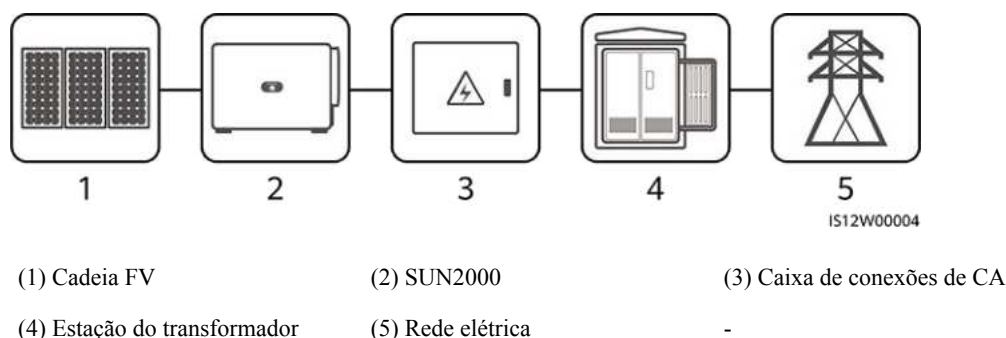
Figura 2-3 Conexão de rede
