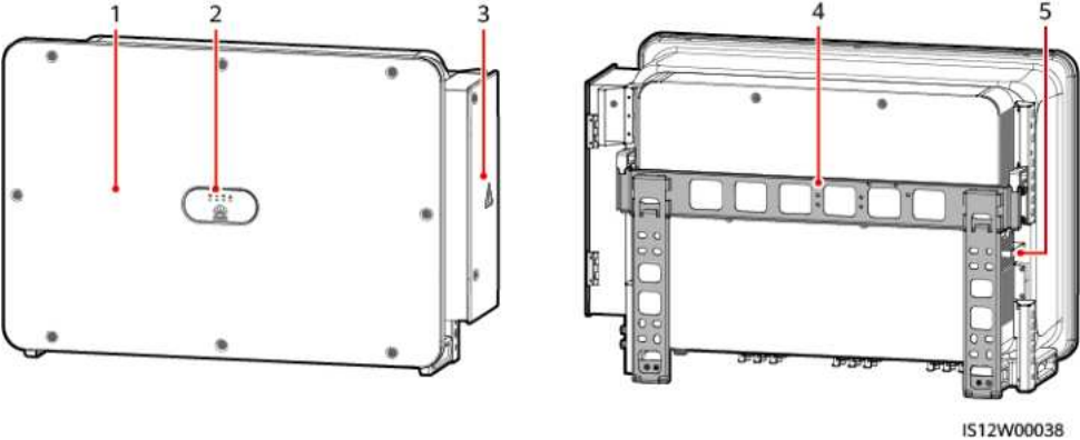
Figura 2-5 Vista frontal
