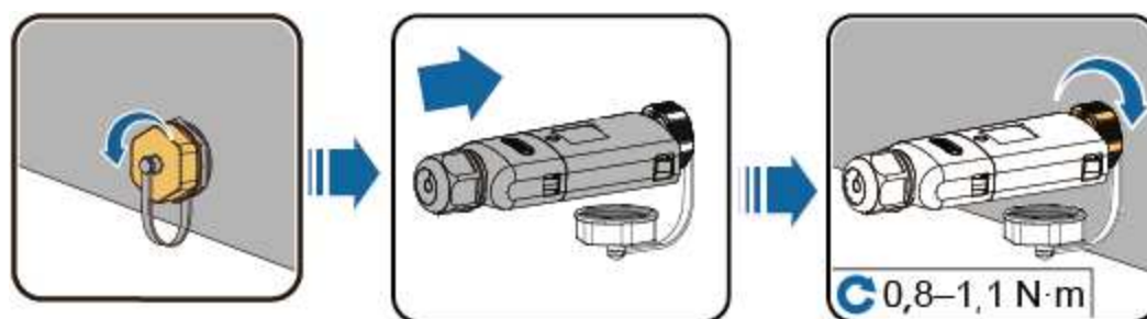
Figura 5-36 Instalação do Smart Dongle WLAN-FE (SDongleA-05 para o cenário de comunicação por WLAN)
