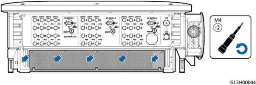
Figura 8-1 Removendo a placa defletora do orifício de entrada de ar
