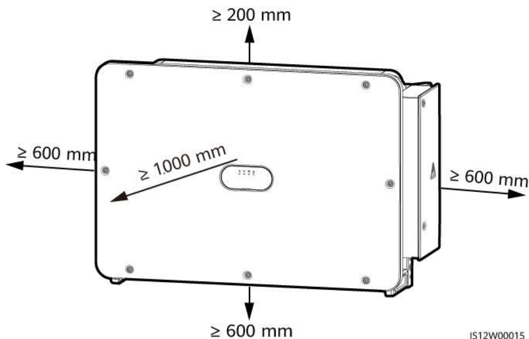
Figura 4-3 Folga
