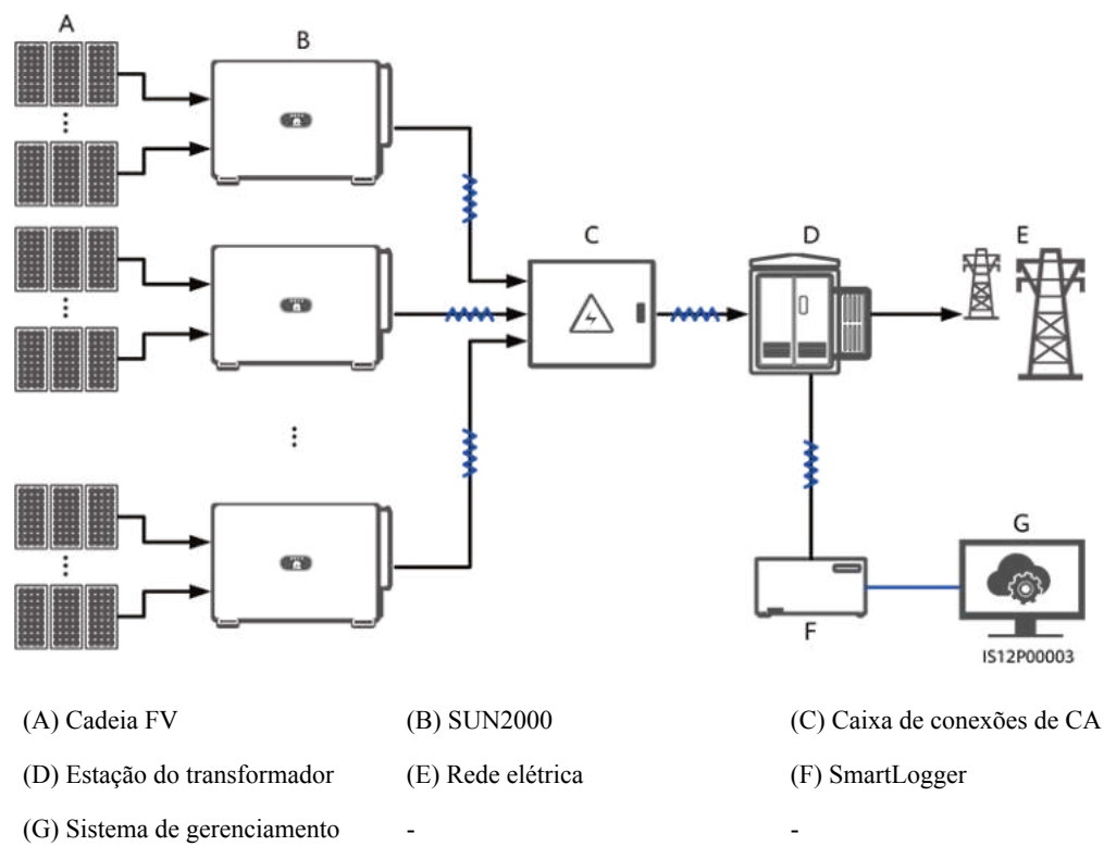
Figura 5-3 Conexão de rede do MBUS (SmartLogger)
