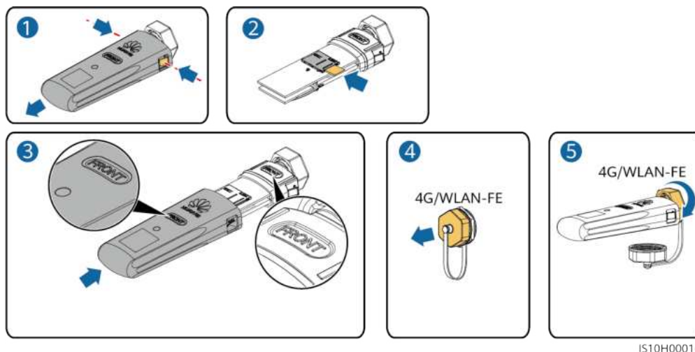
Figura 5-34 Instalação do Smart Dongle 4G (SDongleA-03)
