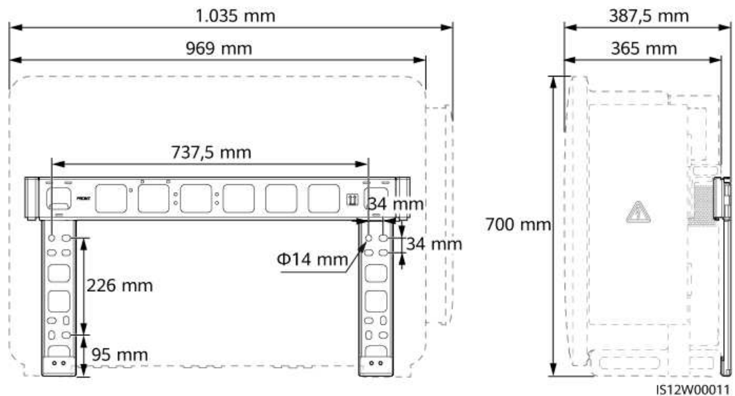
Figura 2-7 Dimensões
