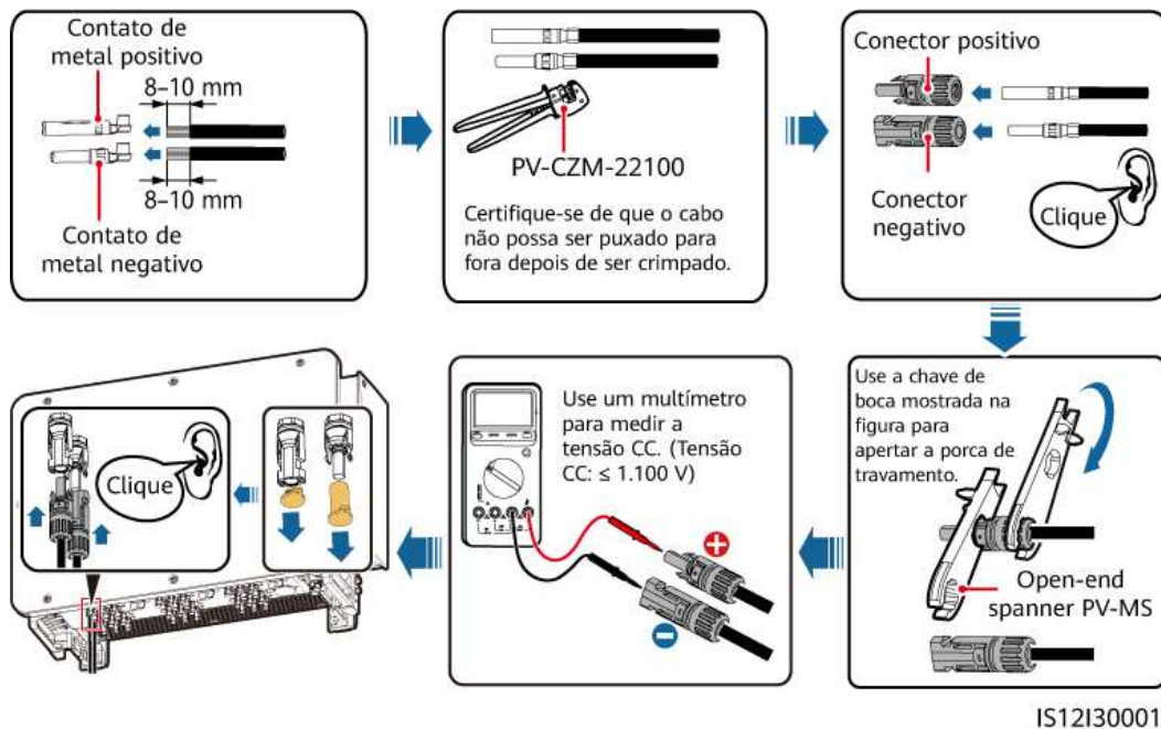
Figura 5-28 Conexão dos cabos de alimentação de entrada CC
