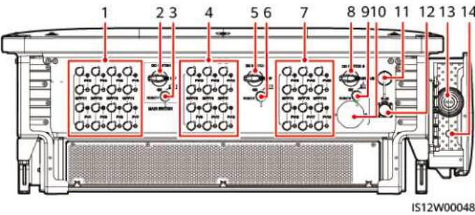
Figura 2-6 Portas
