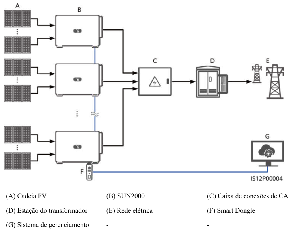
Figura 5-2 Conexão de rede do RS485 (Smart Dongle)
