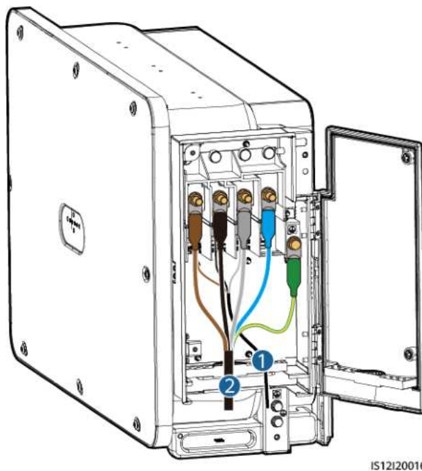
Figura 5-12 Sequência de conexão do cabo
