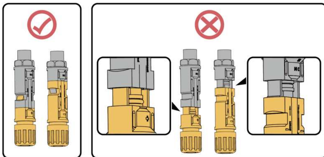
Figura 5-29 Conexão do conector
