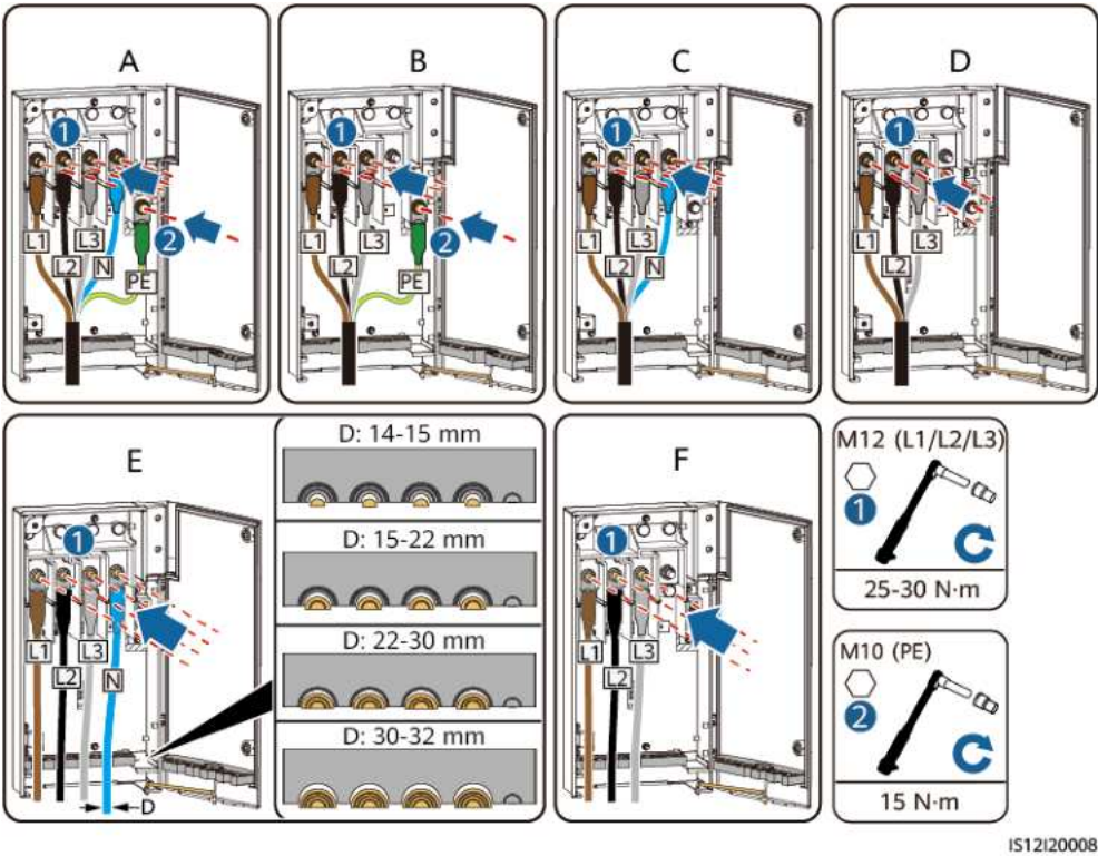
Figura 5-17 Diagrama de conexão
